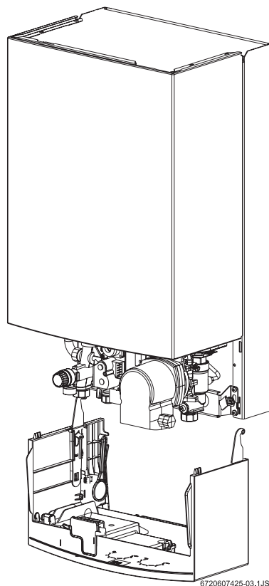
Rys. 12 Demontaż panelu sterującego.
