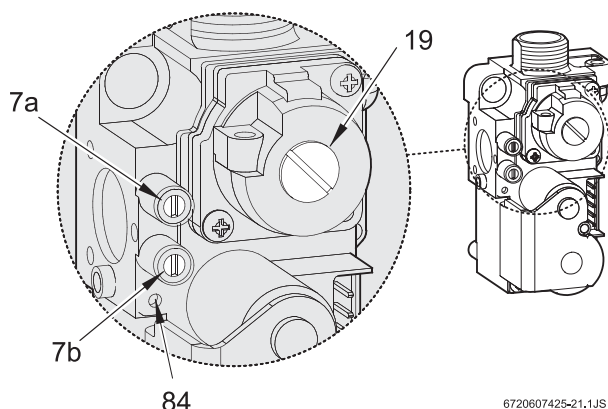
Rys. 31 Armatura gazowa
