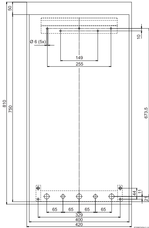
Rys. 8 Szyna + płyta montażowa
