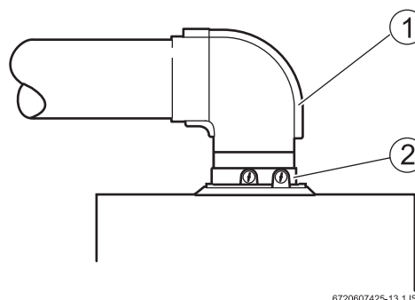
Rys. 14 Umocowanie kolanka rury odprowadzania spalin przy użyciu zacisku
