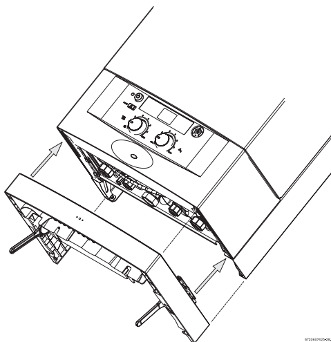
Rys. 17 Ułożenie szuflady
