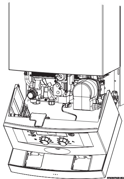
Rys. 30 Pozycja serwisowa
