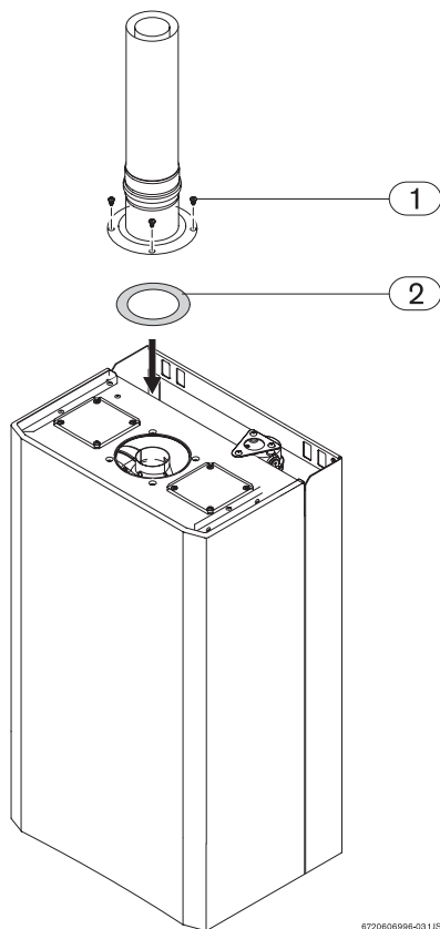
Rys. 15 Montaż kryzy dławiącej
