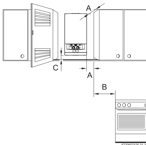
Rys. 7 Minimalne odległości
