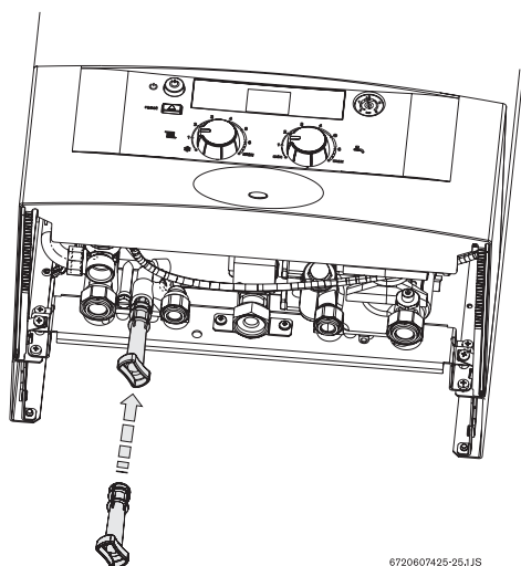
Rys. 18 Uchwyt do napełniania
