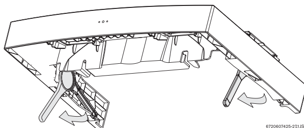
Rys. 16 Uchwyty mocujące
