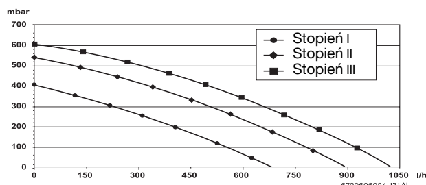
Rys. 6 Charakterystyka pompy
