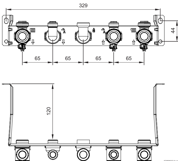
Rys. 9 Płyta montażowa
