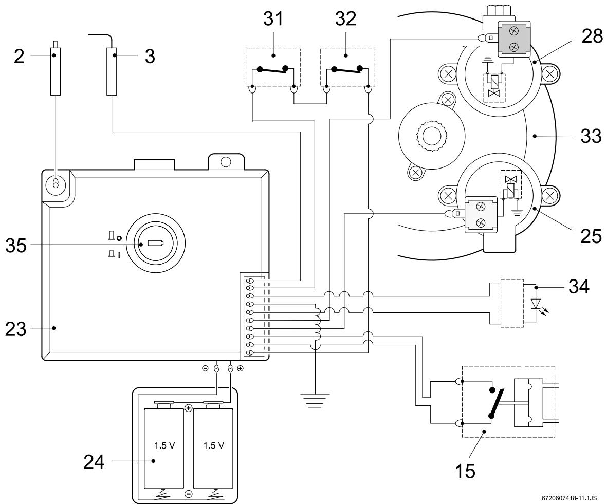
Rys. 3 Schemat instalacji elektrycznej
