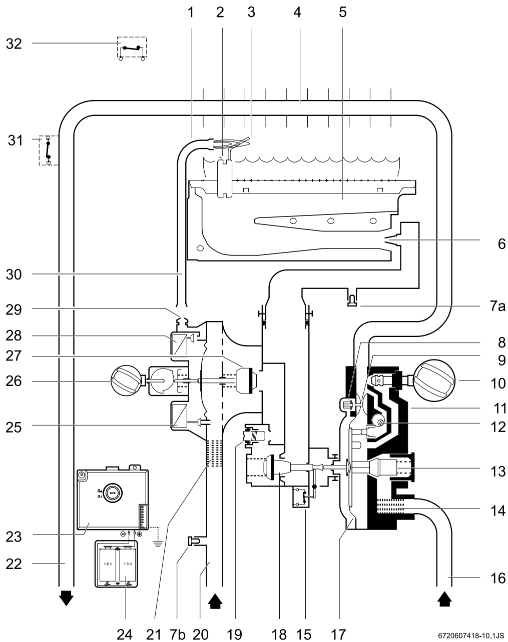
Rys. 2 Schemat działania
