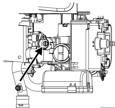
Rys. 14 Śruba do ustawiania maksymalnego natężenia przepływu gazu
