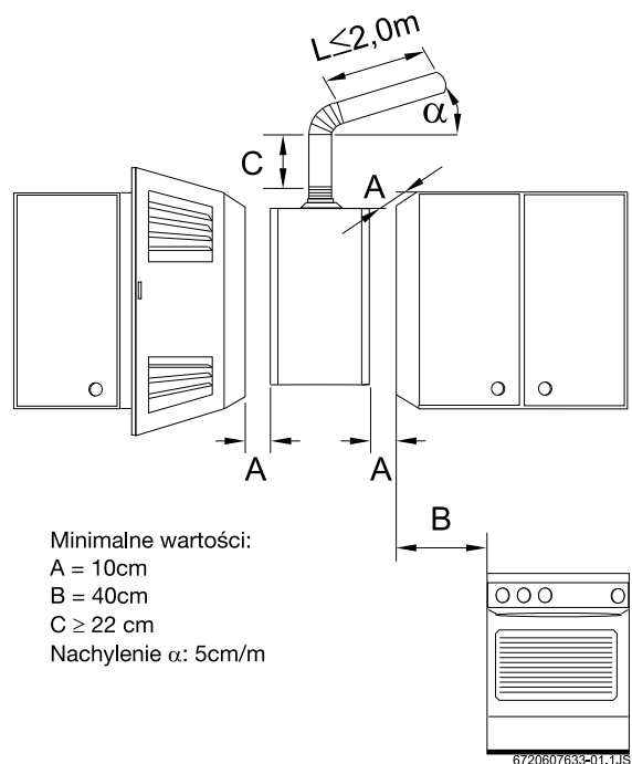
Rys. 4 Minimalne odległości
