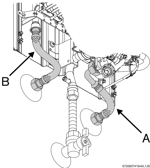
Rys. 5 Podłączenie wody
