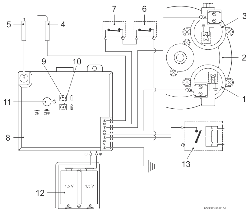
Rys.3 Schemat instalacji elektrycznej
