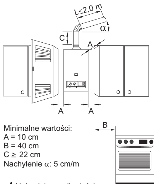
Rys. 4 Najmniejsze odległości przy zabudowie grzejnika
